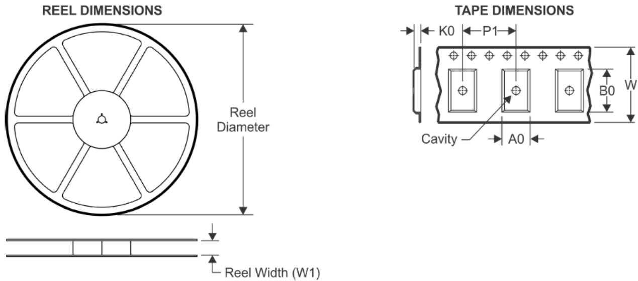
图 34: 载带尺寸图
