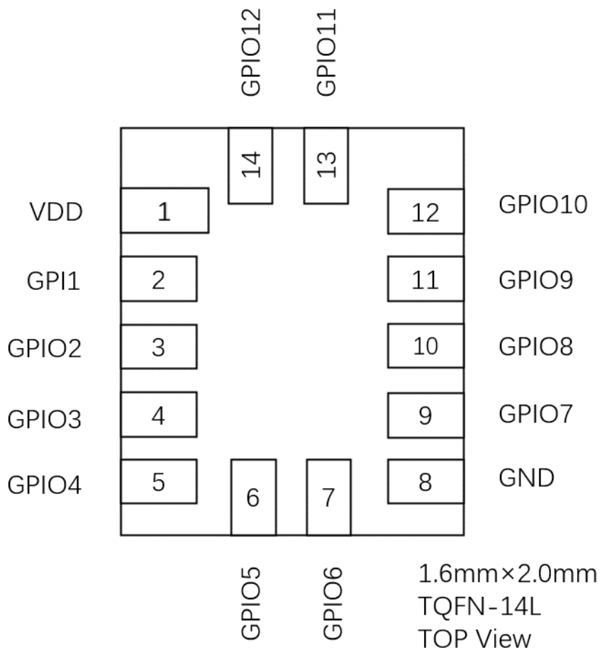
图 2: TQFN-14-L (TOP View)
