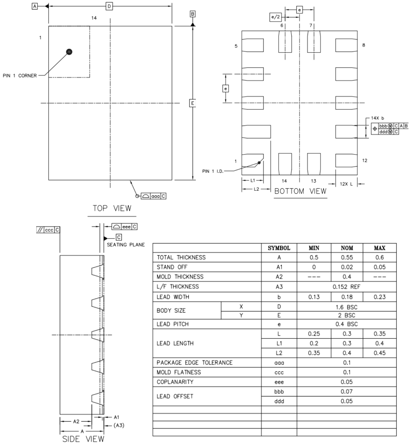
图 33: 封装轮廓图
